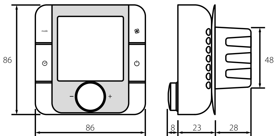
Dimensions hors-tout du CVCPA30
