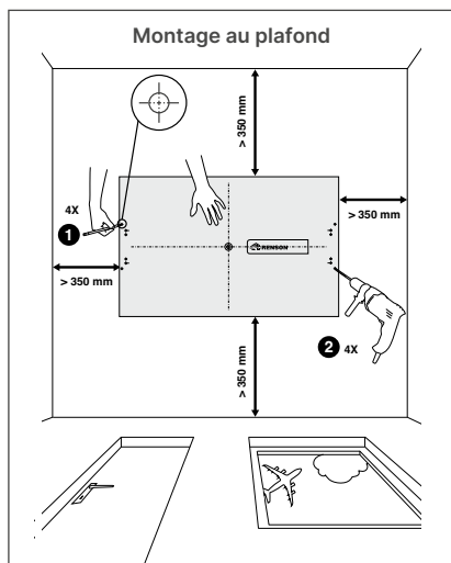
Montage au plafond avec QuickFix – Position dans la pièce (unité en mm) – Configuration des trous de l'équerre QuickFix.
