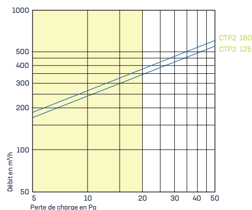
Prise d'air
