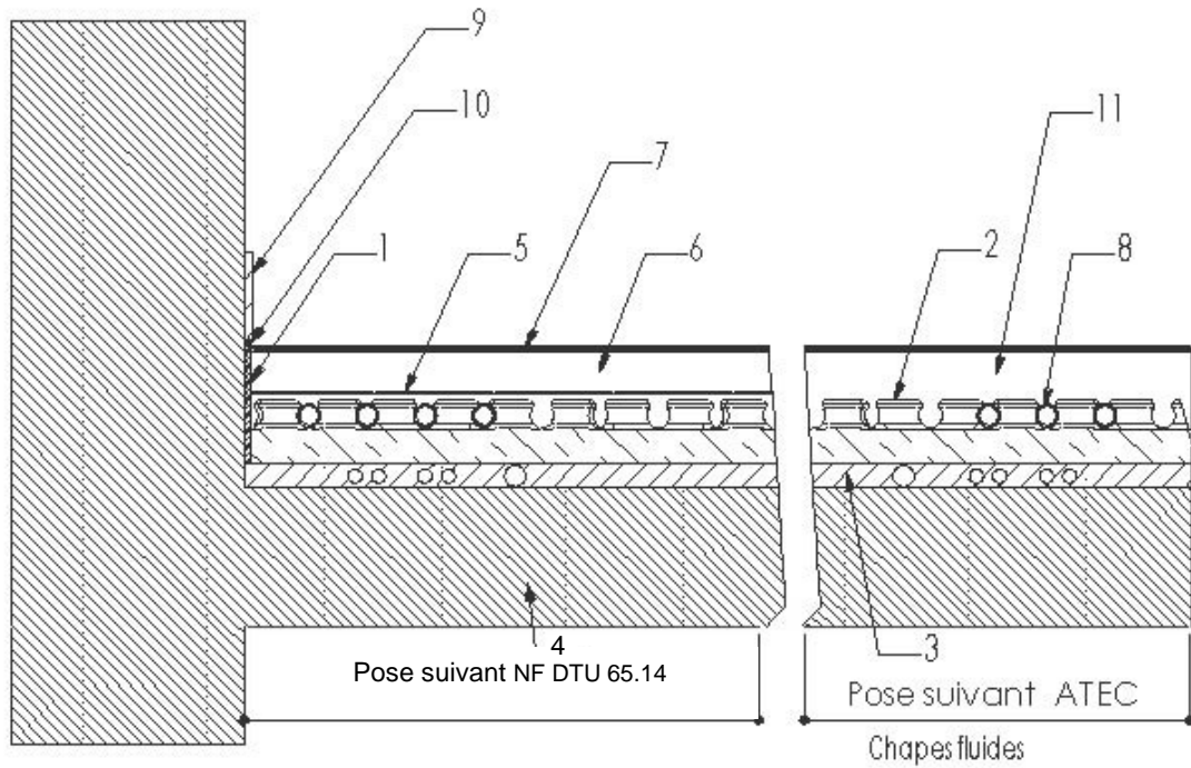
Figure 1 (a) – Dalles à plots isolantes sur ravaillage éventuel en pose désolidarisée isolée
