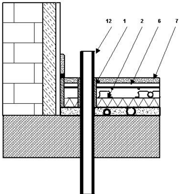
Figure 3 – Cas d'une canalisation verticale avec point fixe passant dans un fourreau ou une gaine en pose désolidarisée
